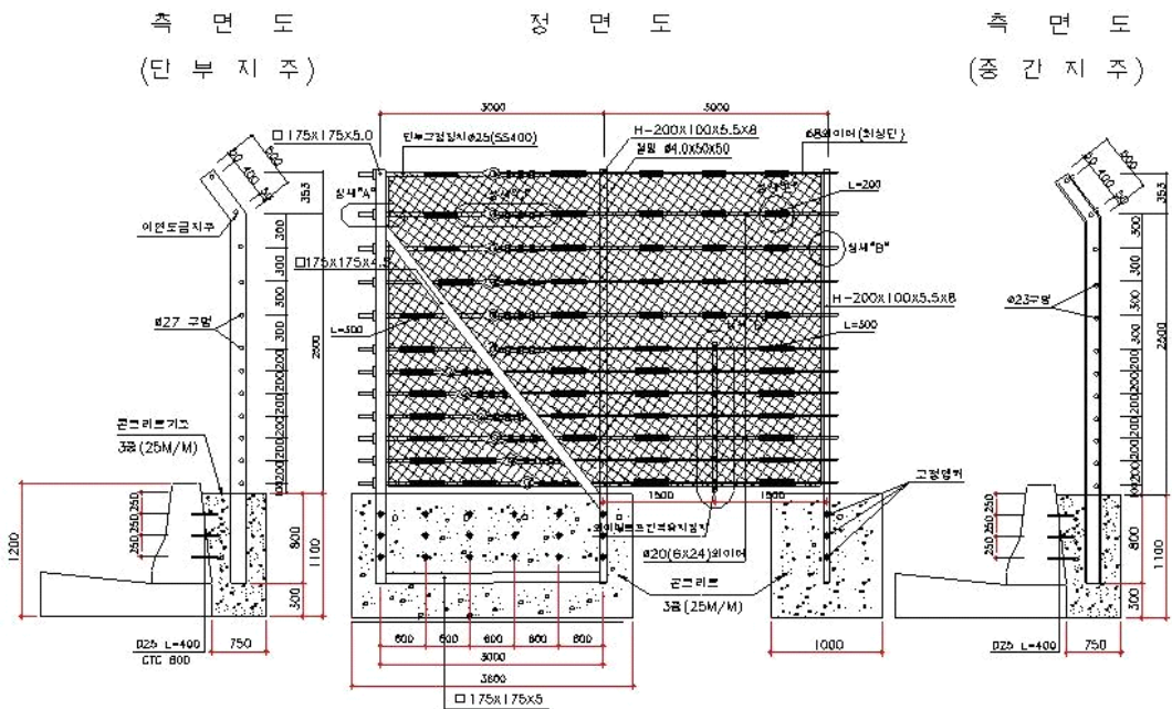
낙석방지울타리 (TYPE-3)
