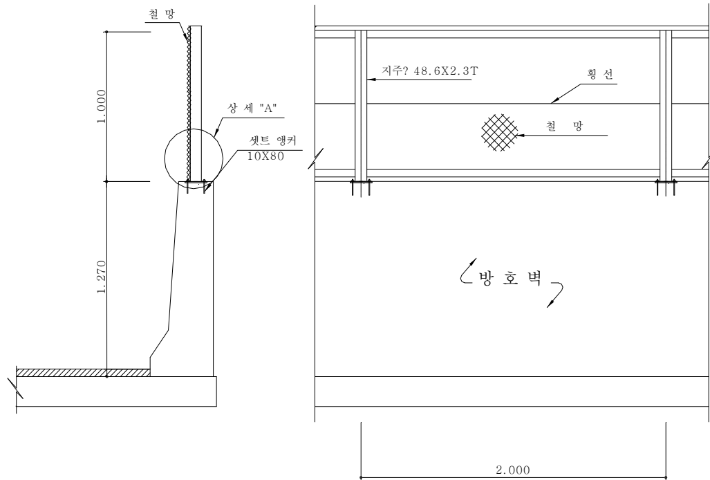
<가드웬스-육교용>
