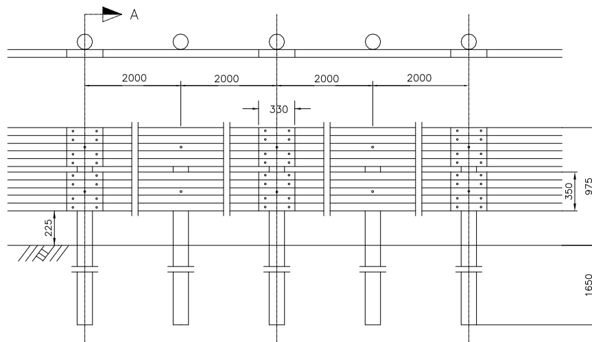
<1단 가드레일>
