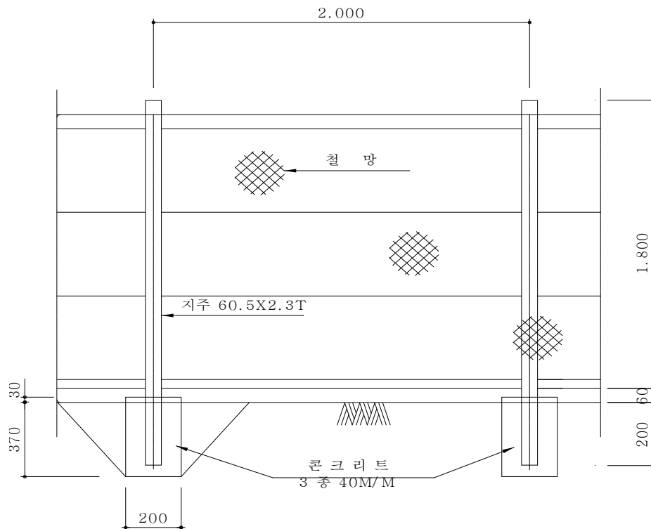
<가드휨스-토공용>
