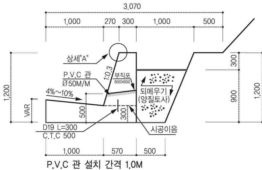
<L형측구 Type - 2>
