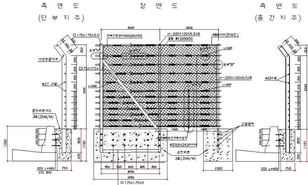
낙석방지울타리 (TYPE-3)
