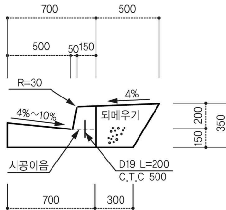
<L형측구 Type-4>
