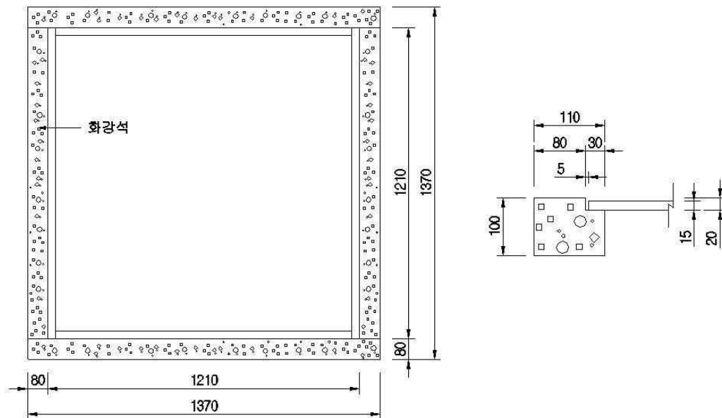
<가로수분(받침틀)>
