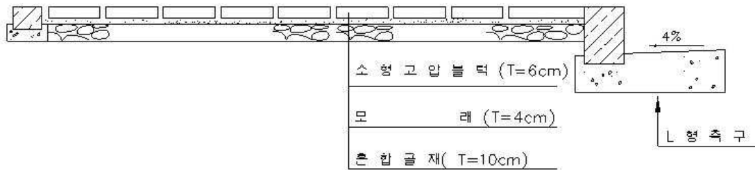
<소형고압블록>
