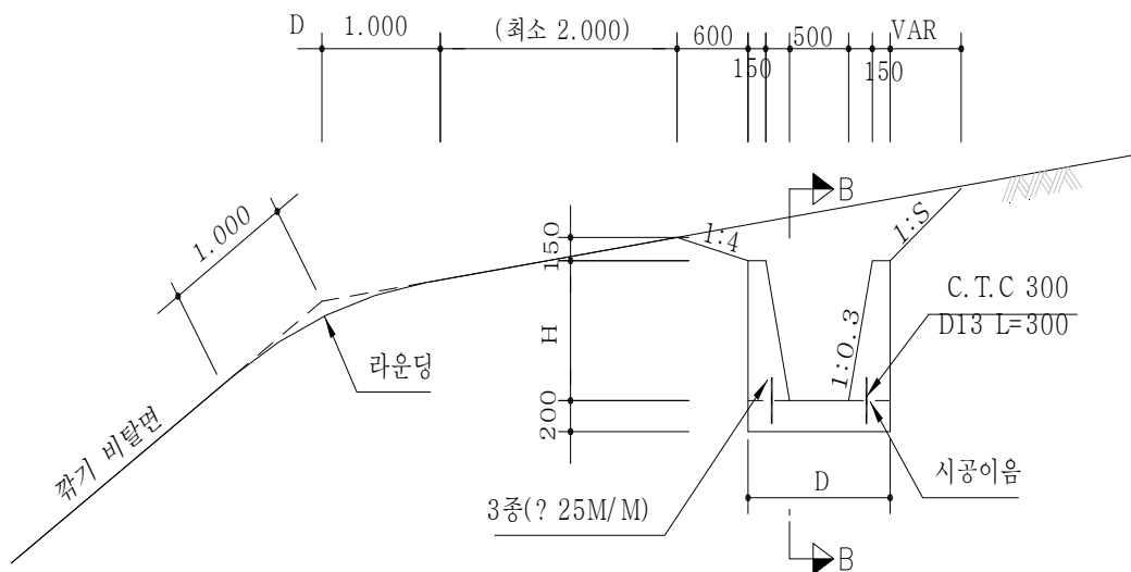
<산마루측구 형식 1,2,3>
