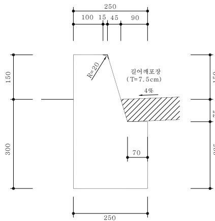
<콘크리트 다이크 Type 1-1>
