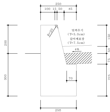
<콘크리트 다이크 Type 1-2>
